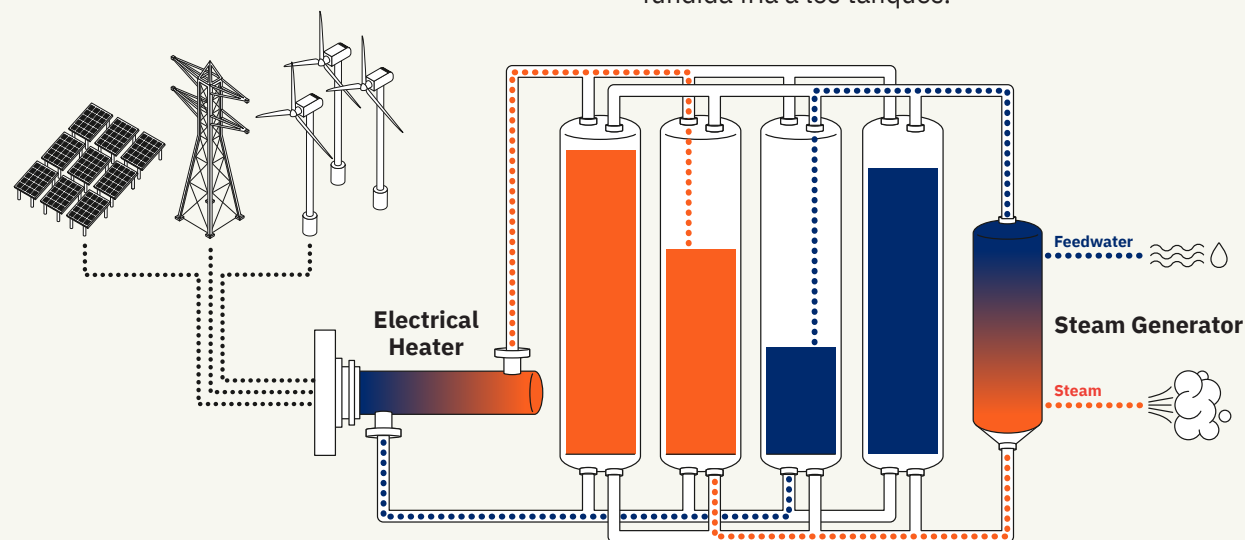
Fig. 1: Proceso de carga y descarga del Heatcube.
