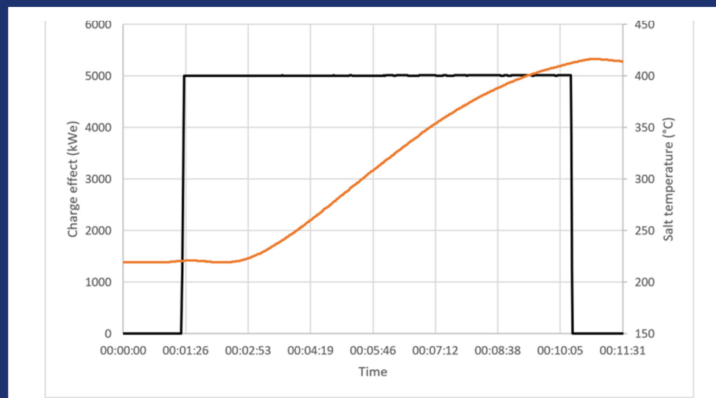
Fig. 4: Representación gráfica de los resultados de las pruebas en el mercado de la energía.
