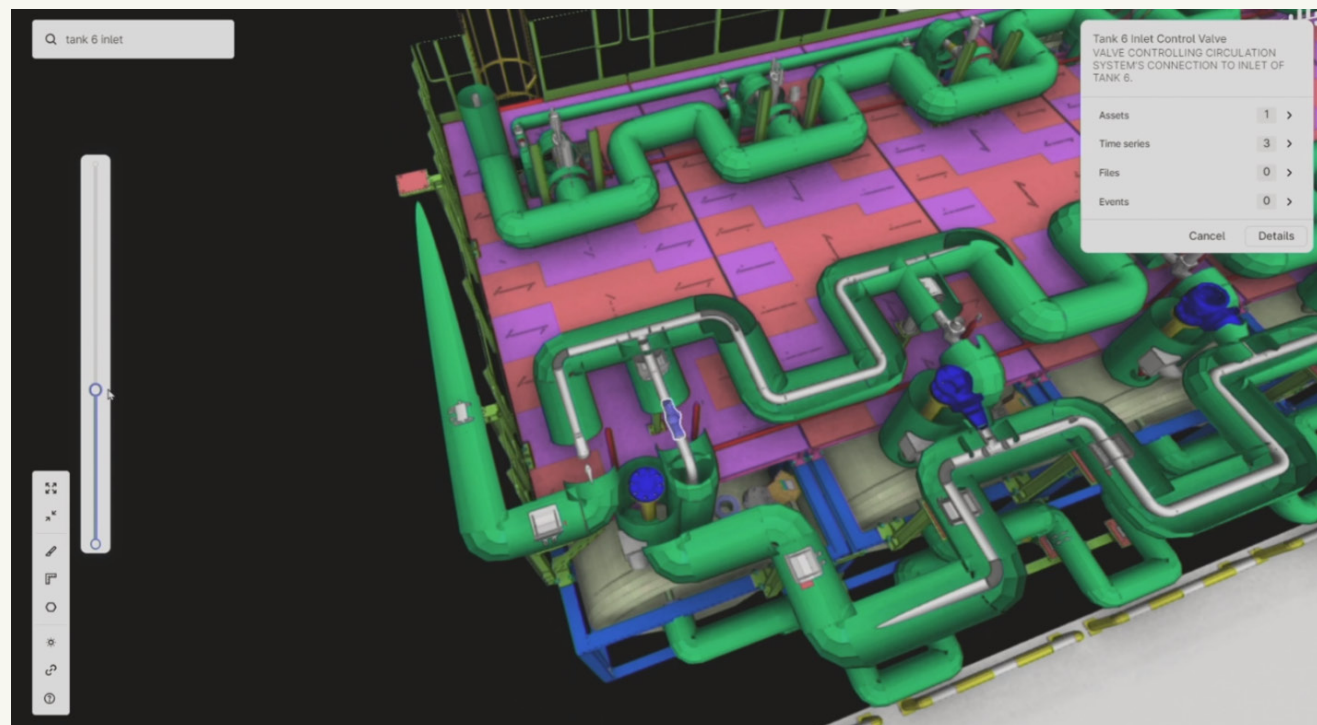
Fig. 5: Heatcube Digital Twin en Norbis Park (Aalborg, Dinamarca).
